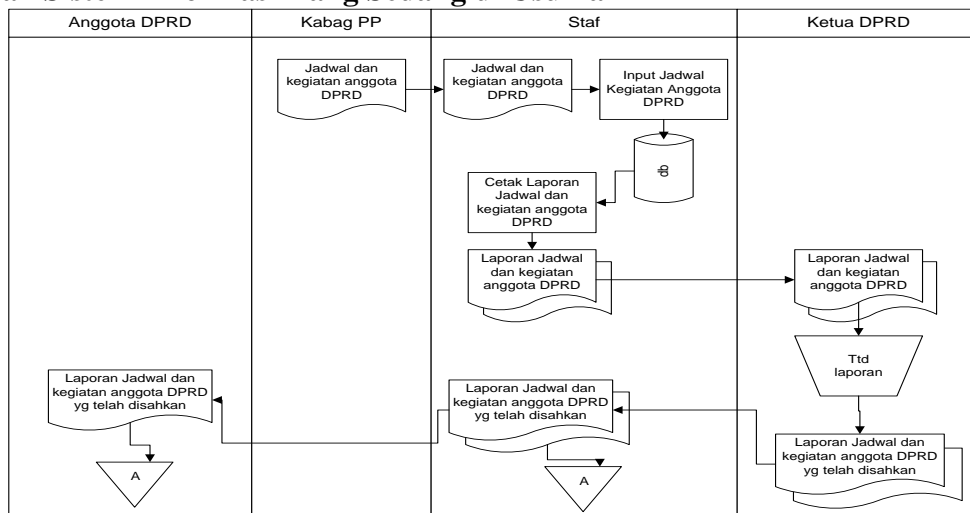
Gambar 3. Aliran Sistem Informasi Yang Sedang di Usulkan
