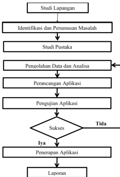
Gambar 1. Rancangan Penelitian
