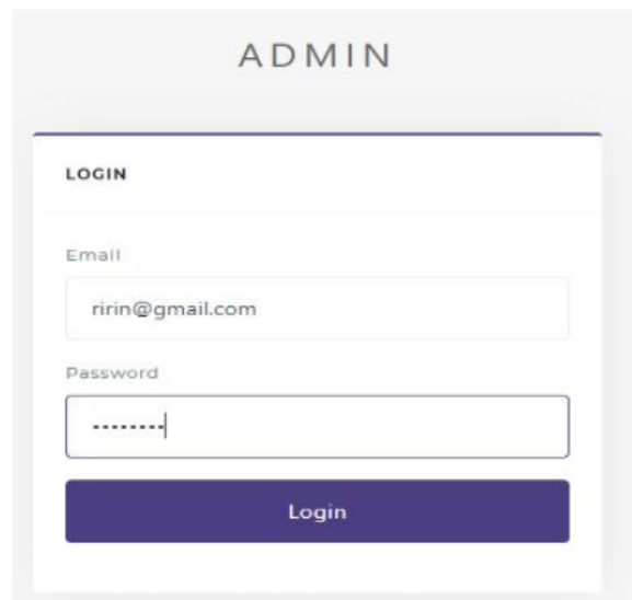
Gambar 4. Halaman Login
