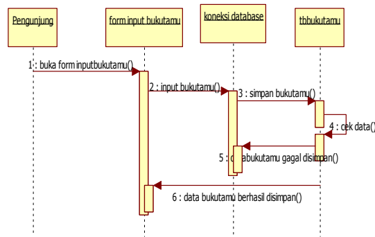
Gambar 4.6 Sequence Diagram Input Bukutamu Pada Pengunjung
