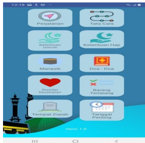
Gambar 10. Halaman Panduan
