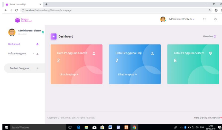
Gambar 6. Halaman Utama
