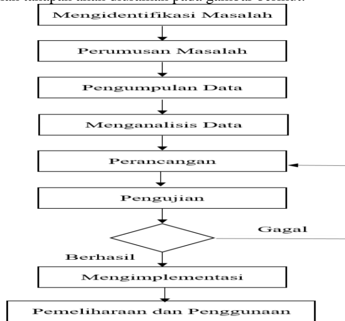
Gambar 1. Rancangan Penelitian
