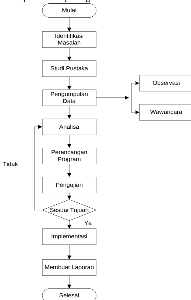
Gambar 1. Rancangan Penelitian
