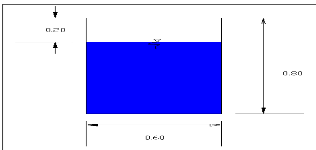
Gambar 4. Dimensi Penampang Saluran Drainase (Sumber : Hasil Perhitungan)
