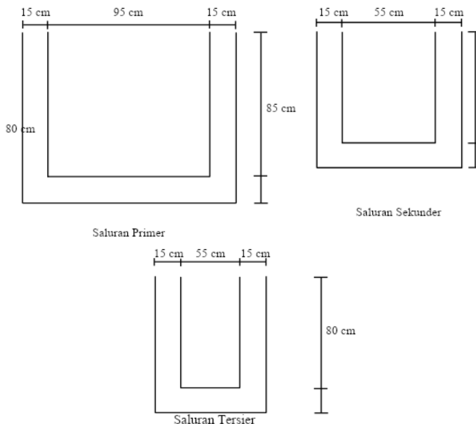
Gambar 2. Dimensi Saluran
