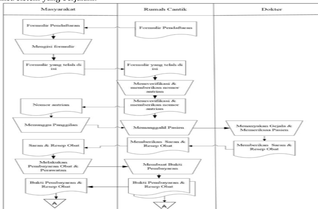
Gambar 1. ASI Yang Sedang Berjalan
