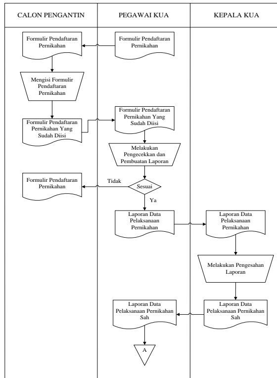
Gambar 1. Analisa Sistem Yang Sedang Berjalan Pada KUA Kecamatan Pangean
