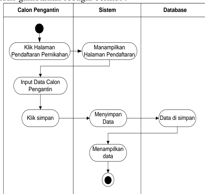
Gambar 6. Activity Diagram Calon Pengantin Melakukan Pendaftaran Pernikahan
