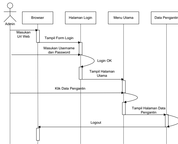
Gambar 7. Sequence Diagram Admin Melihat Data Pengantin
