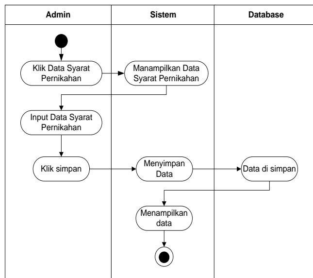
Gambar 4. Activity Diagram Admin Mengelola Syarat Pernikahan
