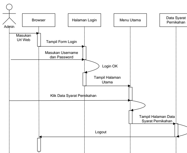
Gambar 8. Sequence Diagram Admin Melihat Data Syarat Pernikahan
