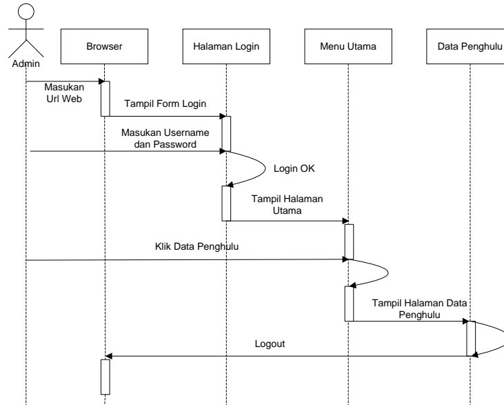
Gambar 9. Sequence Diagram Admin Melihat Data Penghulu
