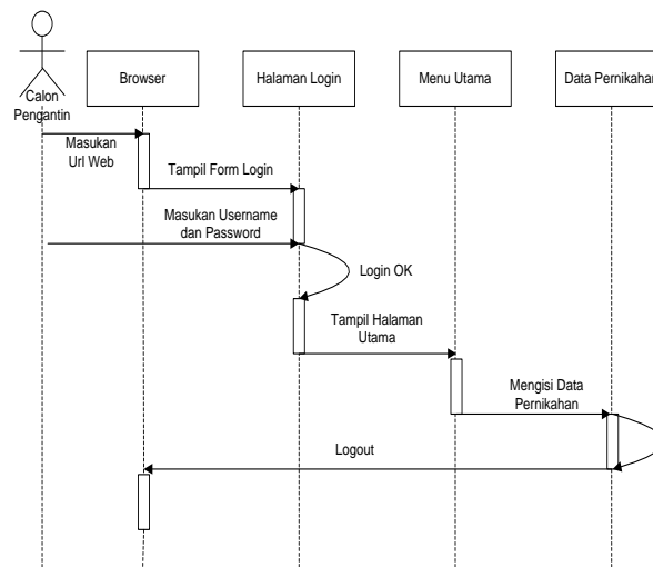
Gambar 10. Sequence Diagram Calon Pengantin Mendaftarkan Pernikahan
