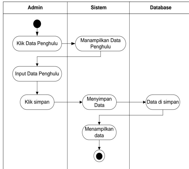
Gambar 5. Activity Diagram Mengelola Data Penghulu
