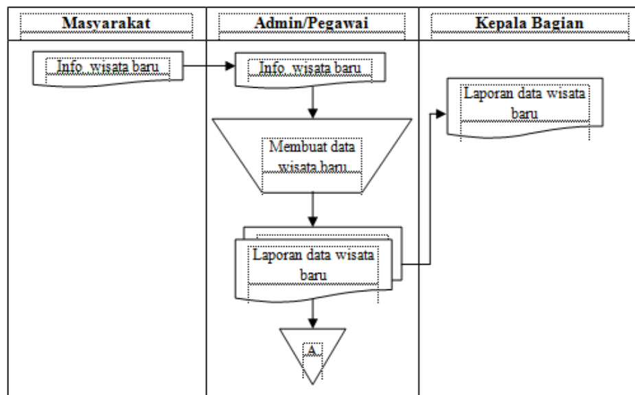
Gambar 2. ASI Yang Sedang Berjalan dari Masyarakat ke Dinas
