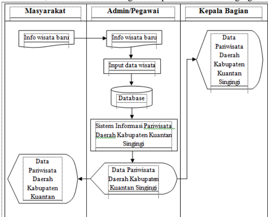
Gambar 4. Aliran Sistem Informasi yang diusulkan
