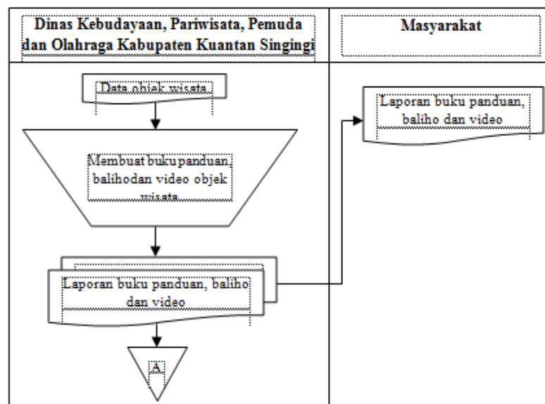
Gambar 3. ASI Yang Sedang Berjalan dari Dinas ke Masyarakat
